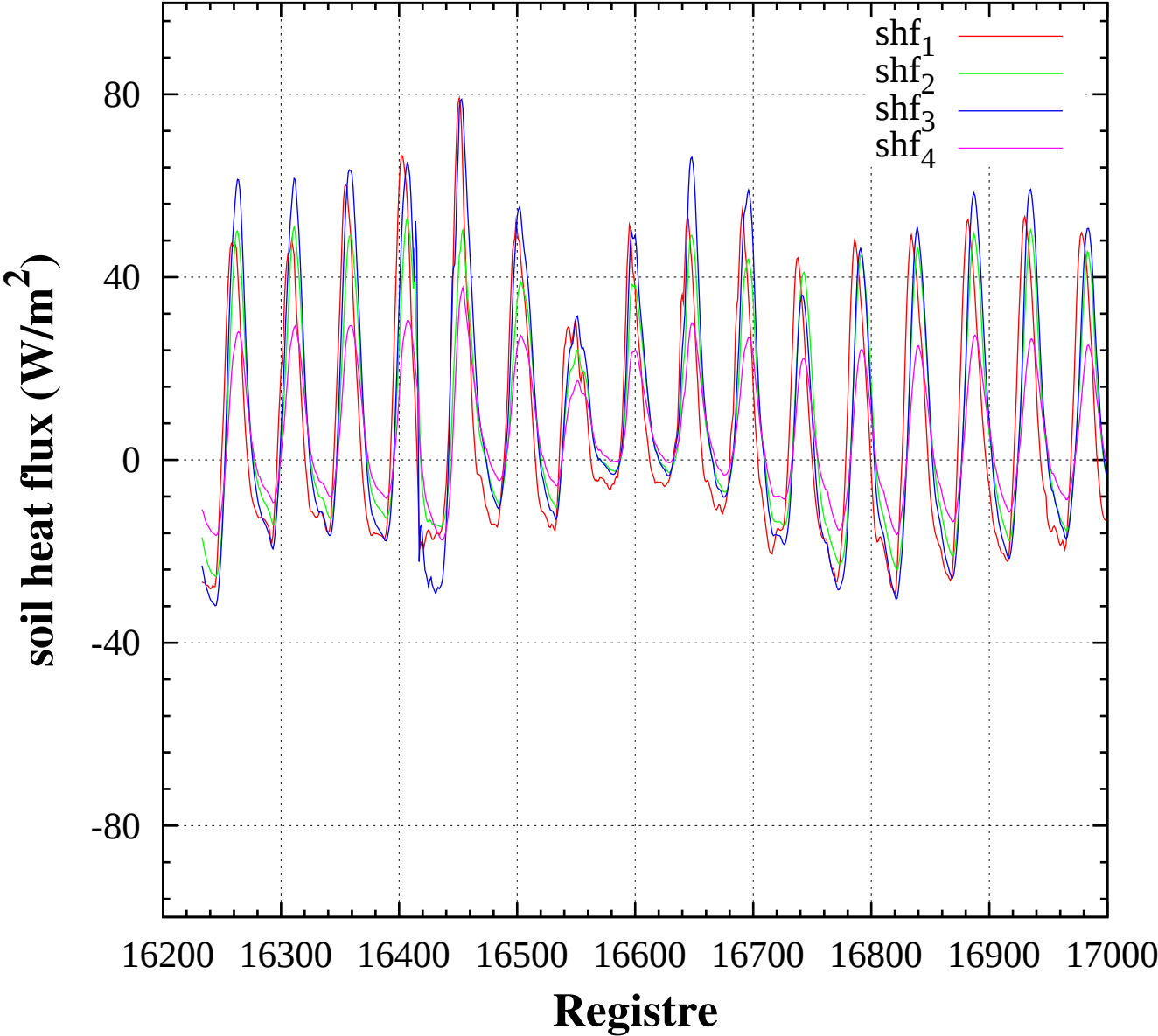
Soil heat flux Raimat 16 a 31 Maig 2009
