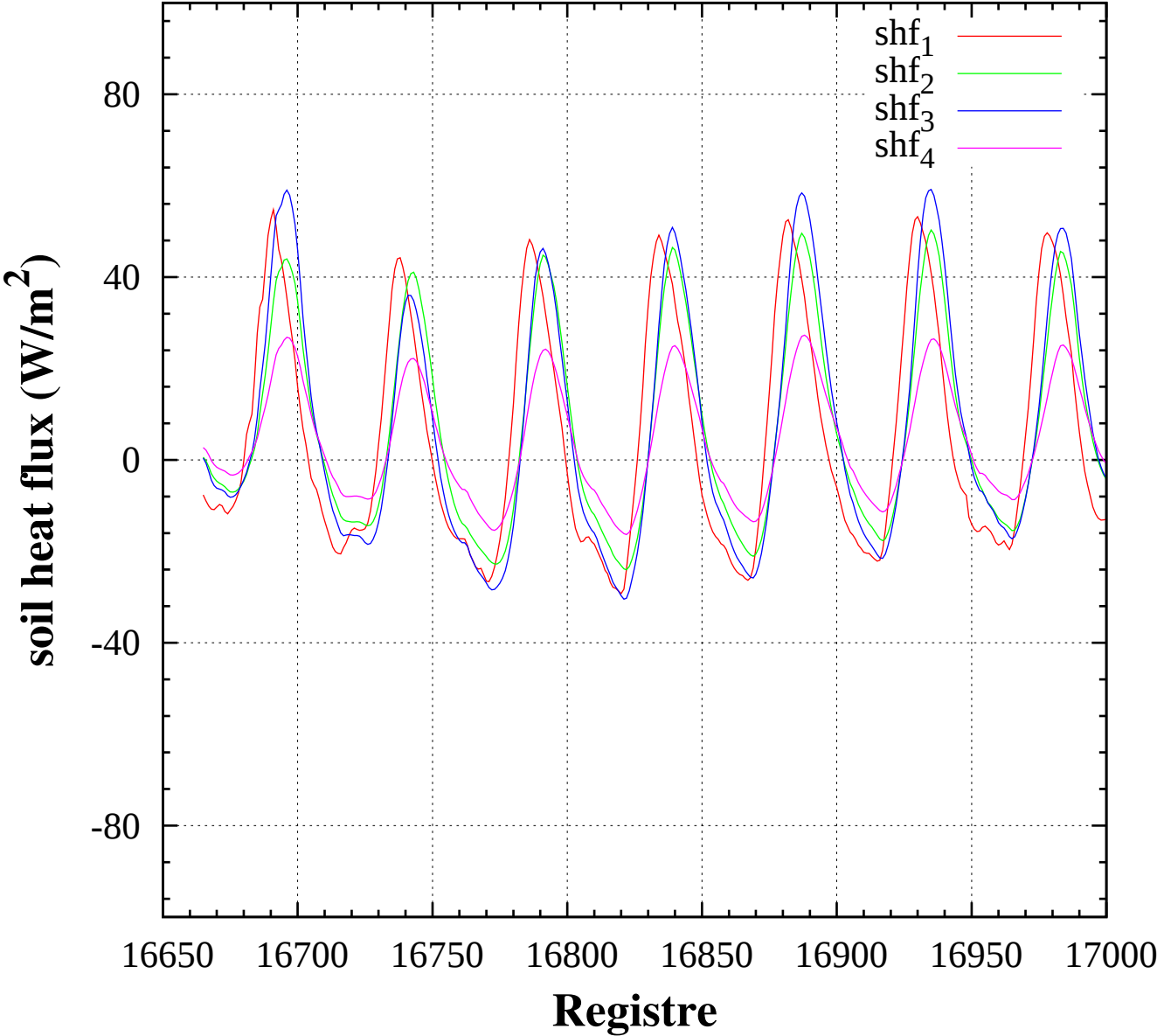
Soil heat flux Raimat 25 a 31 Maig 2009
